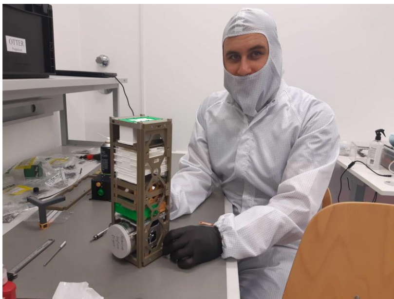
Rysunek 11. Teleskop SOP 1U/65 zintegrowany z platformą satelitarną misji OTTER
