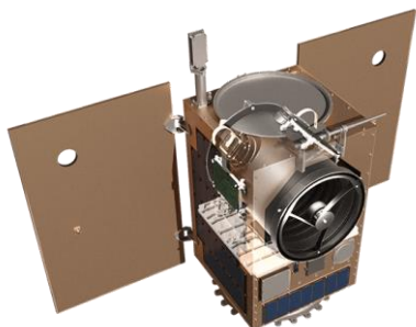
Rysunek 17. Mikrosatelita EagleEye
