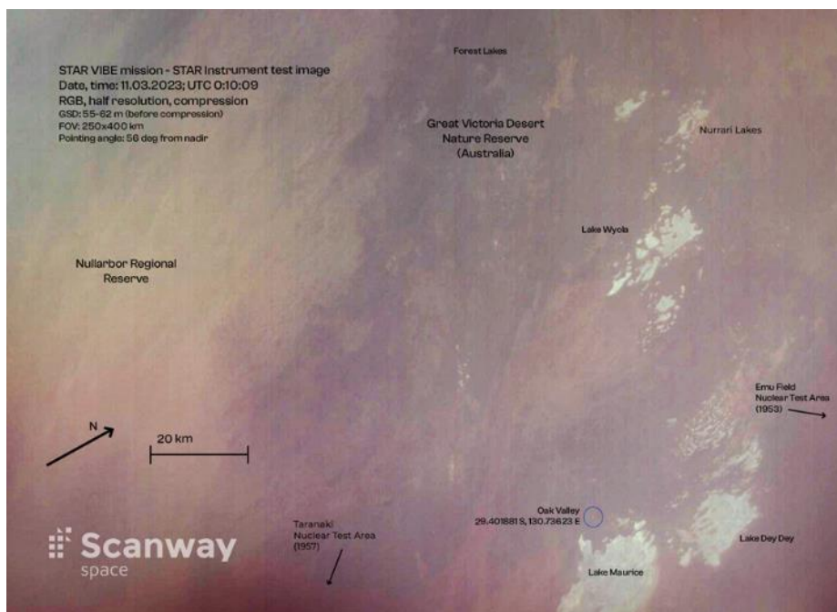
Rysunek 15. Zdjęcie zrobione teleskopem STAR , Australia Południowa (pustynna Nizina Nullarbor)
